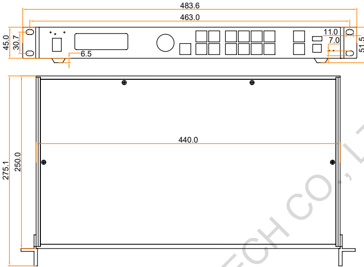
VX4U dimensions (Unit:mm)
